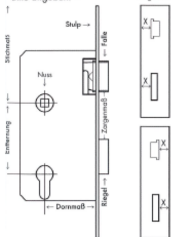
Türprofil - falz
